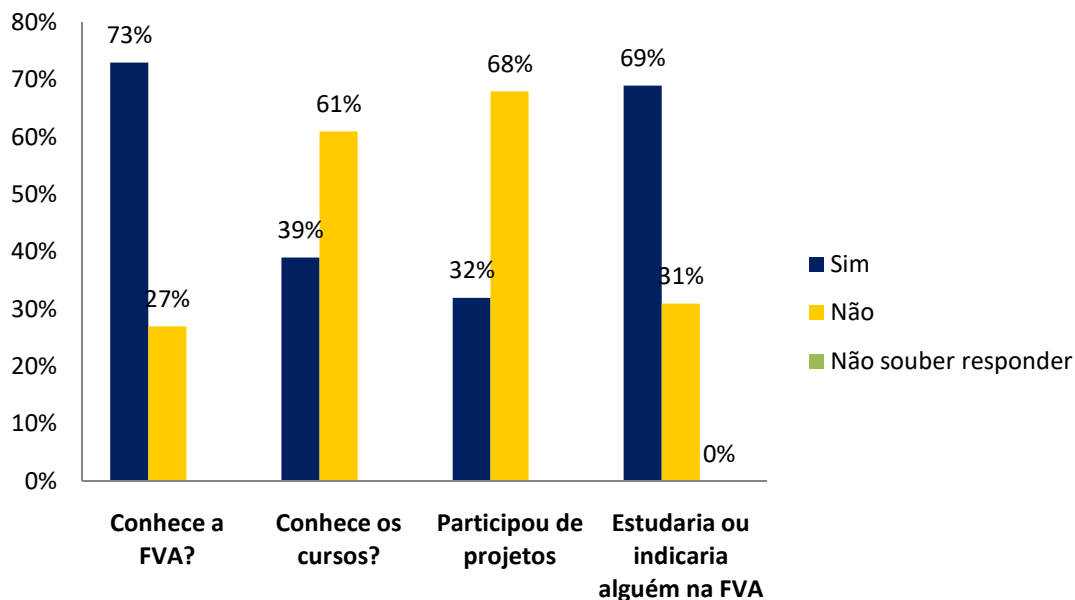
Gráfico 04: Perguntas Gerais.
